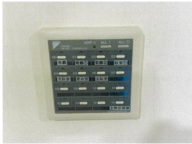
全室空調及全熱交換器總開關面板
